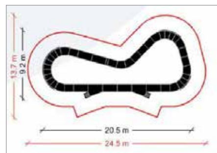
Schéma a rozměrové parametry sestavy
