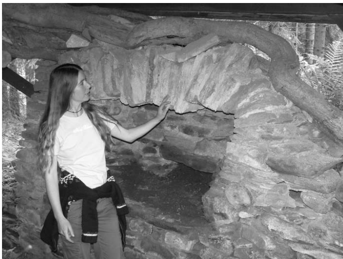
Konzervované zbytky sklářské chladicí pece z 18. století ve Staré hutí I u Podlesí - Vogelsangu u Kašperských Hor (významná památka historie sklářství zkoumaná archeologicky) foto Vladimír Horpeniak
